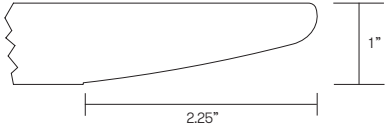
Edge Detail # 38
